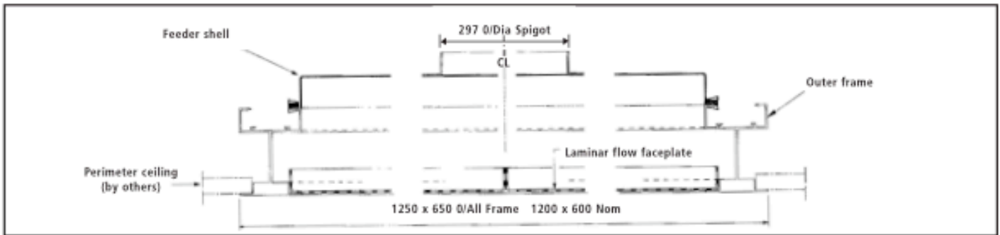
Section through model PAR single panel
