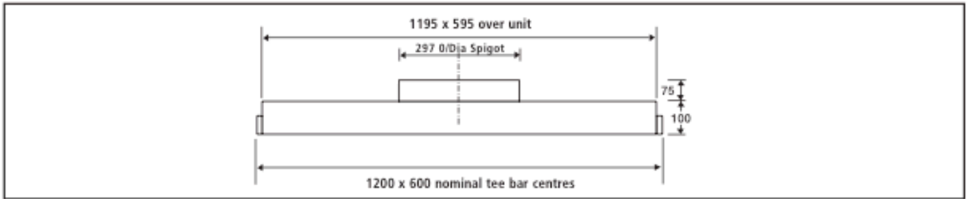
Section through model PAR single panel
